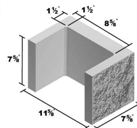
12x8x8 Lintel
