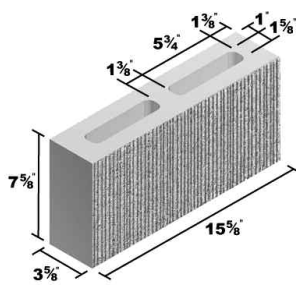
4x8x16 Standard
