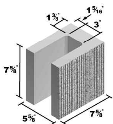
6x8x8 Lintel
