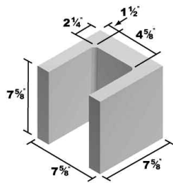
8x8x8 Lintel
