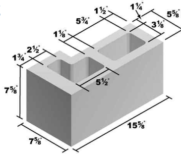
6x8x16 Dogleg
