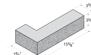
4x4x16x8 L Return
