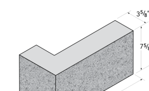
4x8x16x8 L Return
