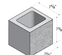
8x8x8 Standard
