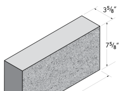
4x8x16 Solid
