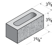
4x4x8 Standard
