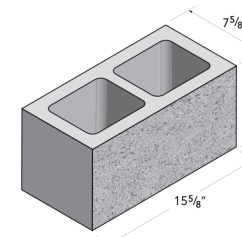
8x8x16 Standard
