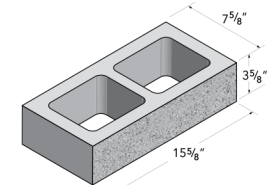
8x4x16 Standard
