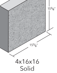
4x16x16 Solid
