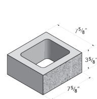
8x4x8 Standard
