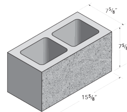
8x8x16 Standard
