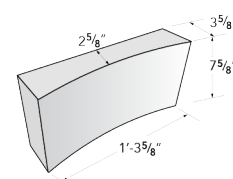
Abri Concave
