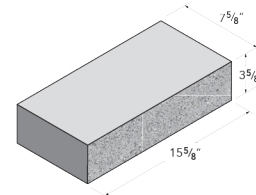
8x4x16 Solid
