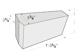
Abri Wedge
