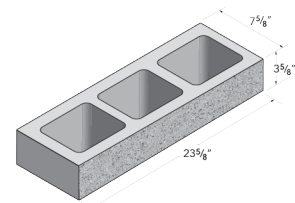
8x4x24 Standard
