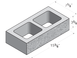
8x4x16 Standard
