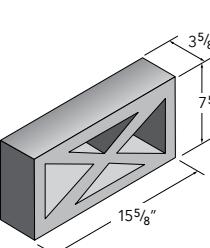
4x8x16
