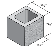
8x8x8 Standard
