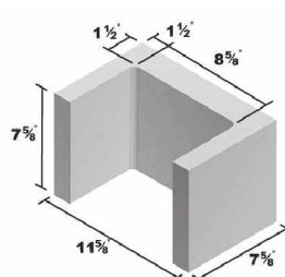
12x8x8 Lintel
