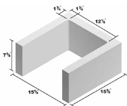
16x8x16 Lintel
