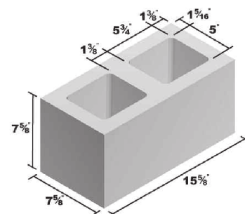
8x8x16 Standard
