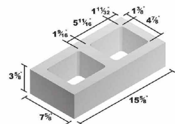
8x4x16 Standard
