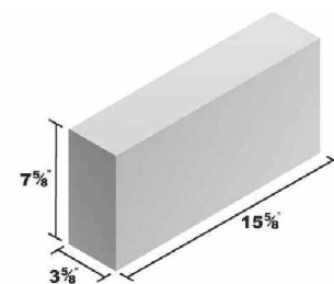
4x8x16 Solid
