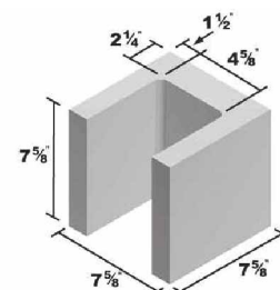
8x8x8 Lintel
