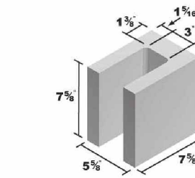
6x8x8 Lintel
