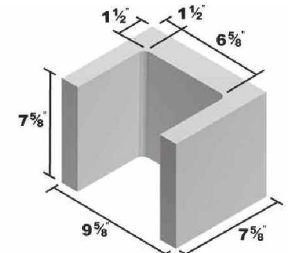
10x8x8 Lintel
