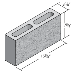
4X8X16 STANDARD
