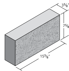
4X8X16 SOLID
