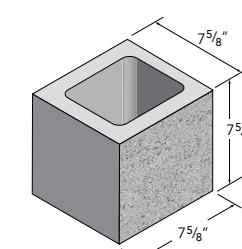
8X8X8 HALF
