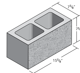
8X8X16 STANDARD
