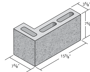
4X8X16 "L" CORNER
